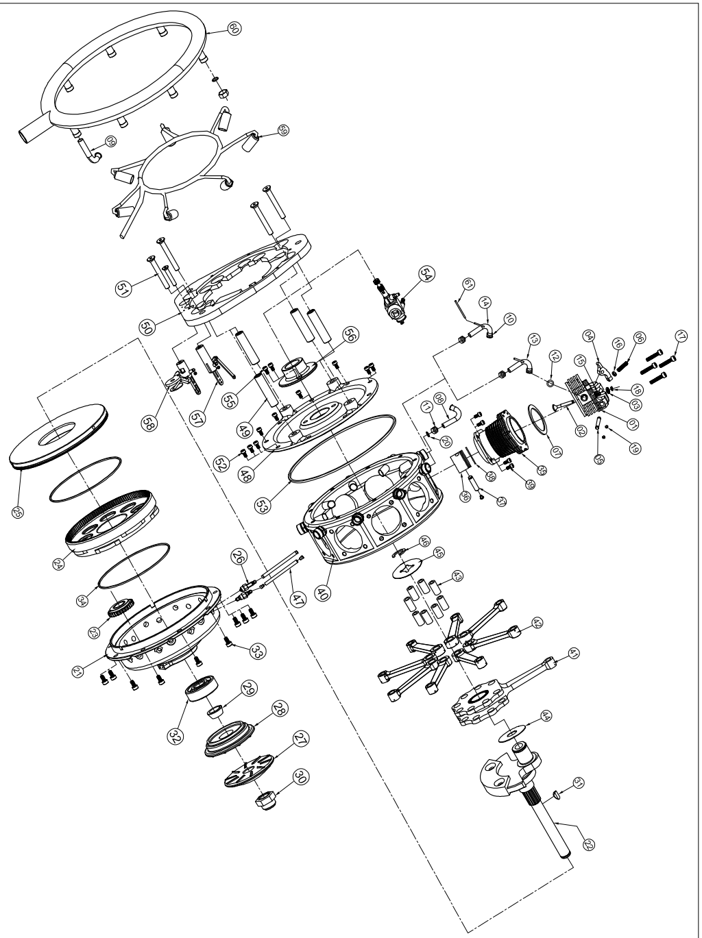
UMS 9-99 RADIAL ENGINE (GLOW) (UMSG409RB099)
