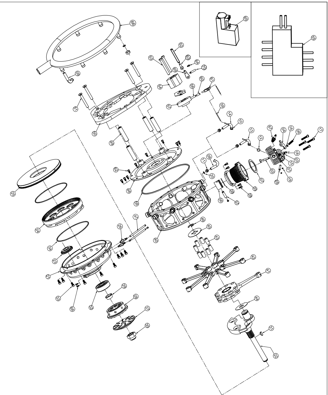
UMS 9-115 RADIAL ENGINE (PETROL) (UMSB409RB115)
